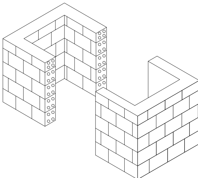
PERPECTIVA DA BASE ANTES DA EXECUÇÃO DA LAJE
