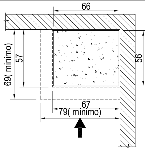
PLANTA KIT DE CANTO POSIÇÃO DIREITO (D) FRENTE LADO MAIOR
