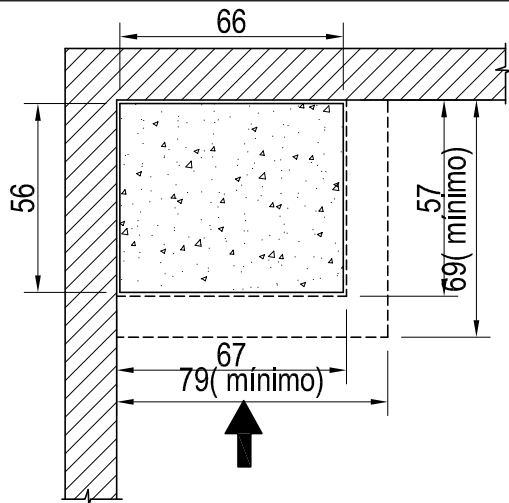
PLANTA KIT DE CANTO POSIÇÃO ESQUERDO (E) FRENTE LADO MAIOR
