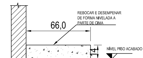
CORTE TRANSVERSAL
