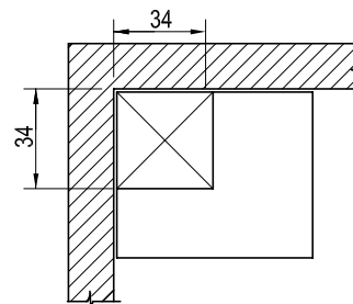
DETALHE DO FURO NA LAJE
