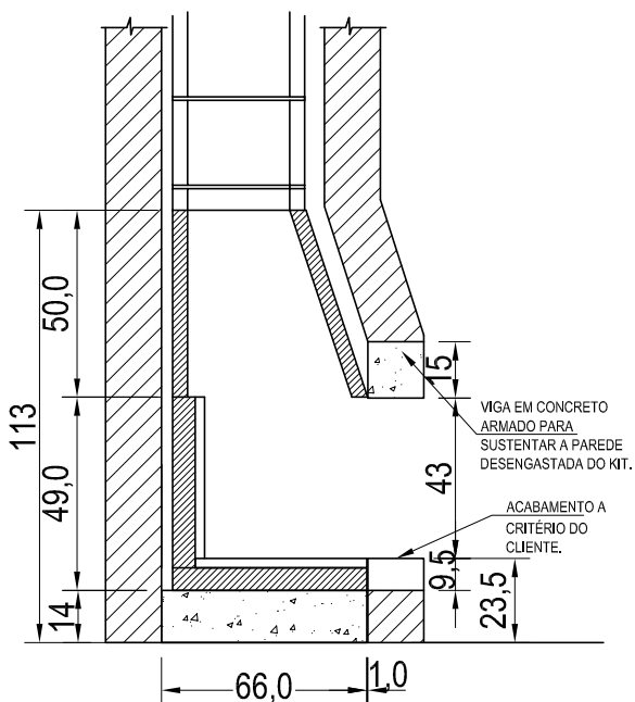
CORTE ACABADO
